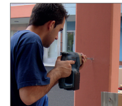
5 Percer les trous à l'aide du marteau perforateur (M10).
